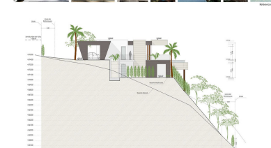
URB. MONTEMAYOR ALTO. PARCELA H5 / east elevation scale 1/150
