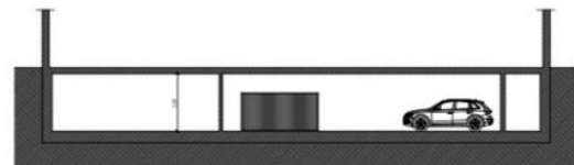
SECCIÓN E-E'
