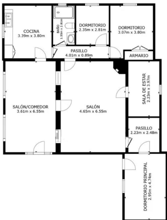
PLANTA
