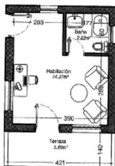
LA CASITA - UPPER FLOOR
