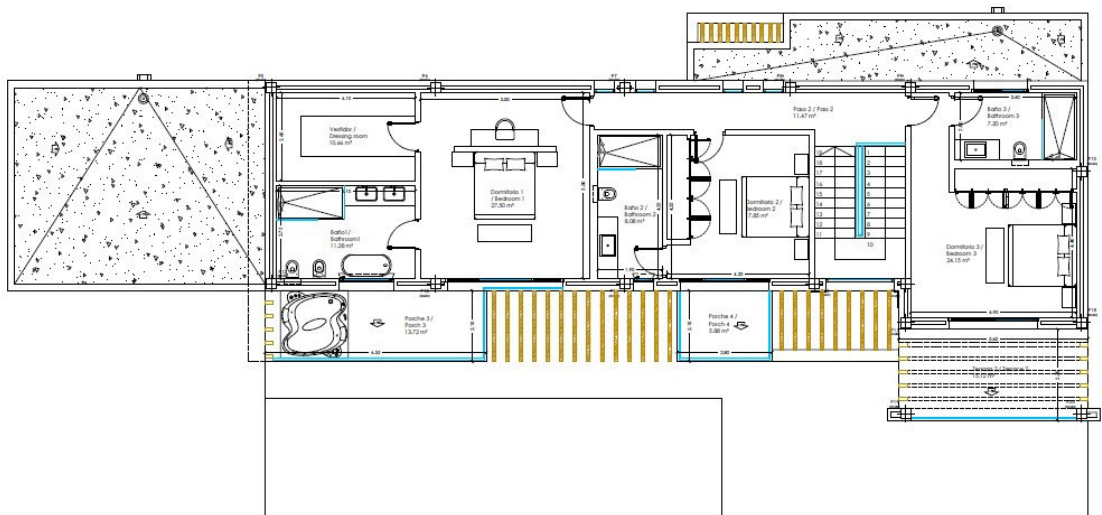
Planta Alta 157.41 m²
