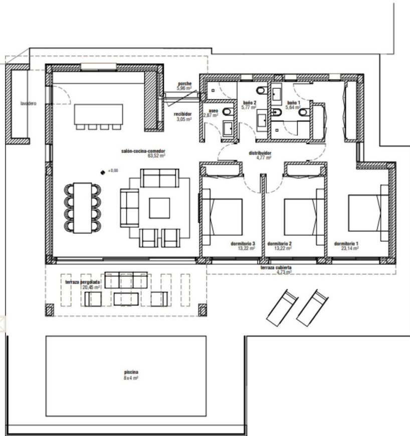
PLANTA BAJA e: 7 : 100
