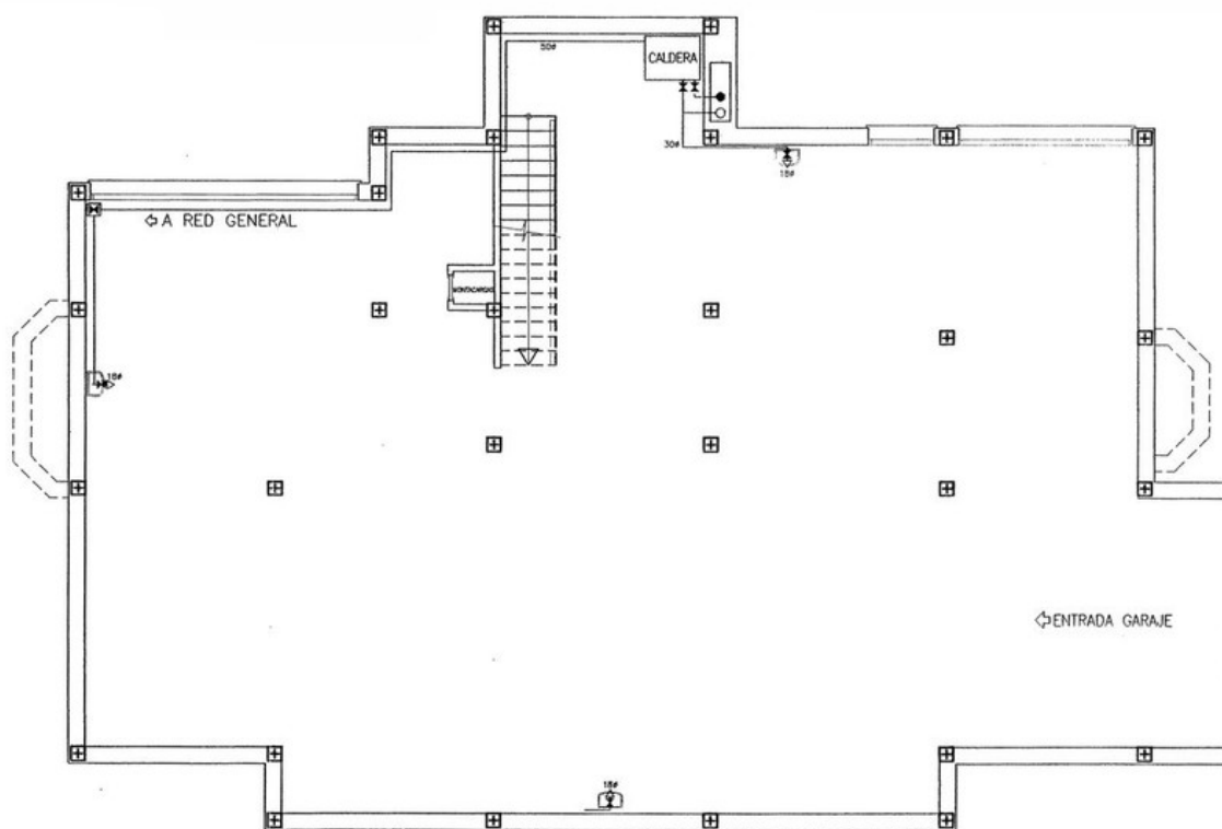
PLANTA SOTANO
