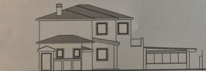
ALZADO NOROESTE
