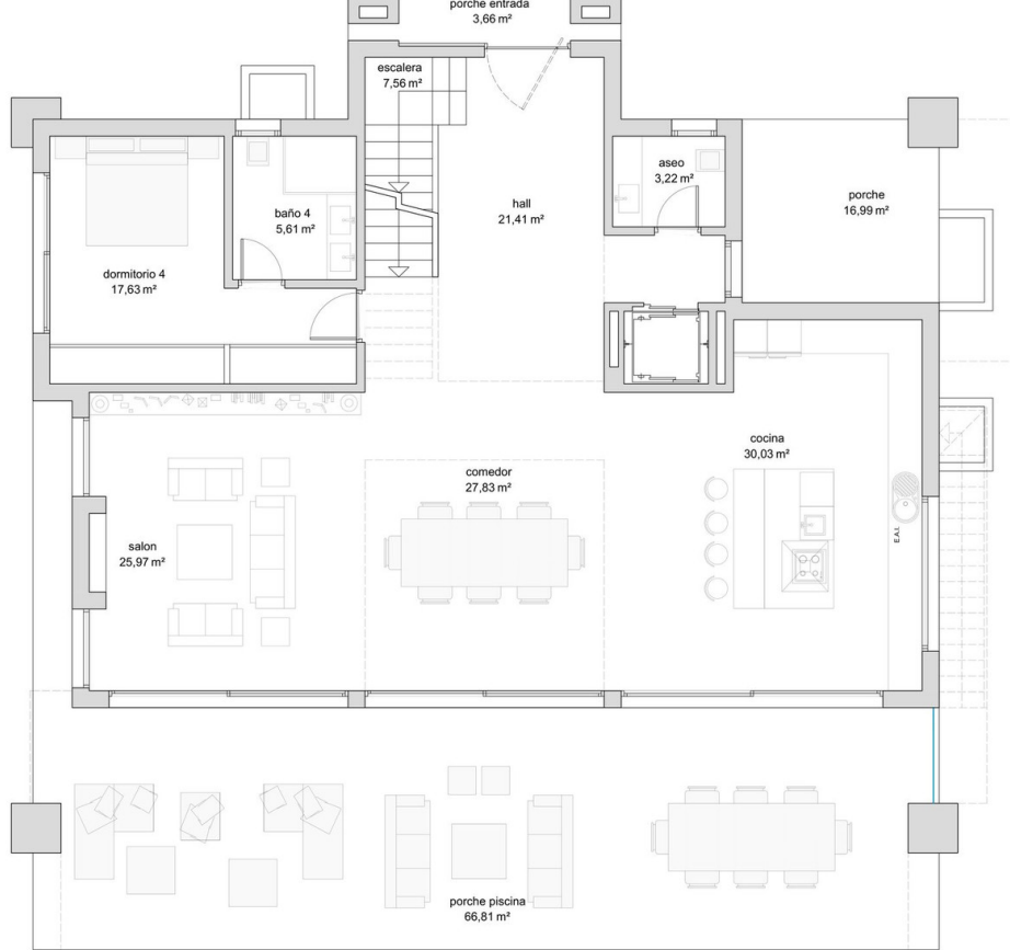
PLANTA BAJA
