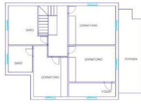
PLANTA ALTA
