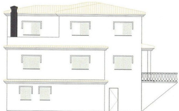
ALZADO 4
