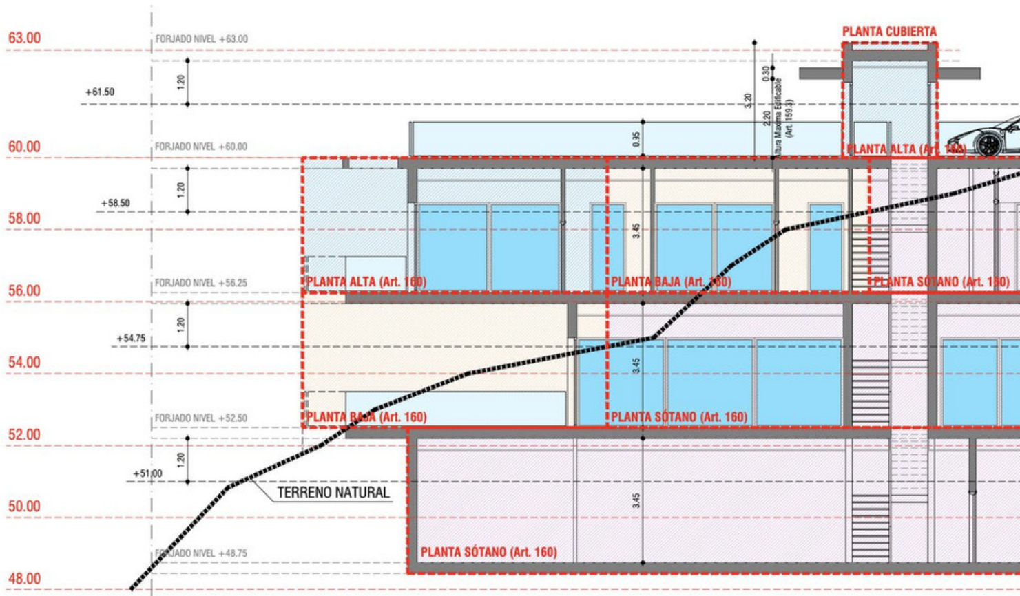
SECCIÓN
