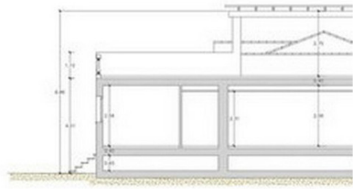
SECCION 8-8
