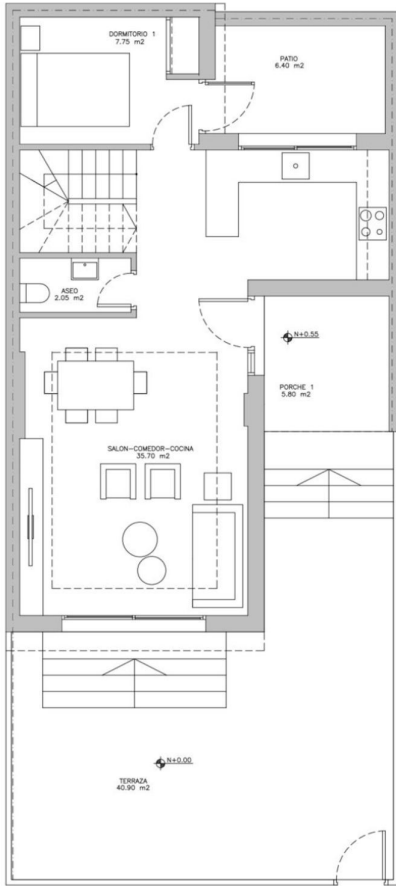
PLANTA BAJA REFORMADO Sup.Construida: 58.20 m 2 Sup.Porche: 9.80 m 2
