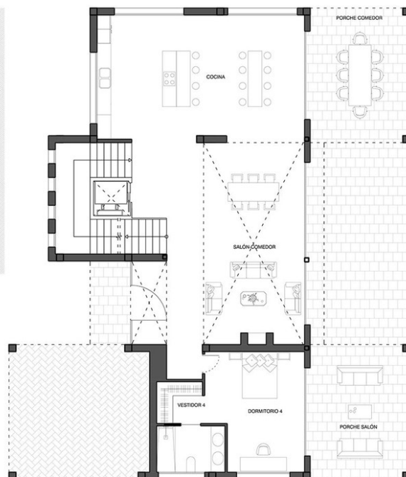
PLANTA BAJA
