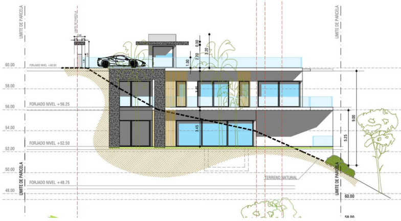
ALZADO SUR
