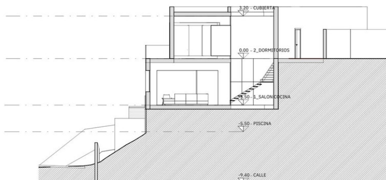
1 SECCIÓN ESCALERA INTERIOR 100 A100
