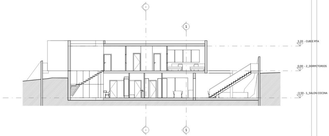
1 SECCIÓN ESCALERA INTERIOR 100 A100
