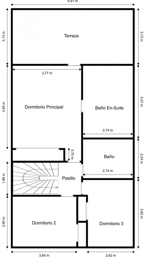
Montevideo Montevideo P1 Plano
