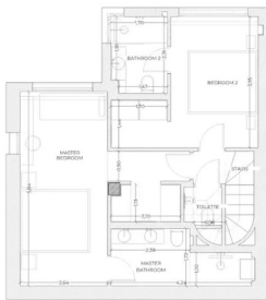
PLANTA -1
