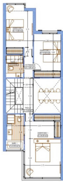
PLANTA PRIMERA
