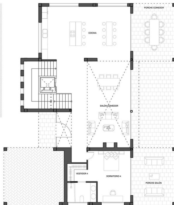
PLANTA BAJA
