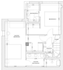
PLANTA -1
