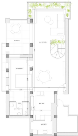
PLANTA BAJA
