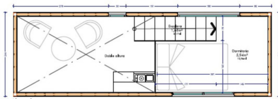
Planta alta
