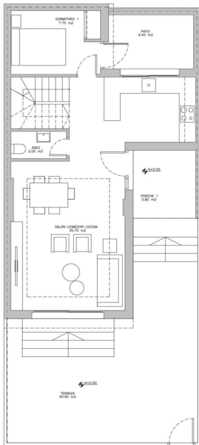
PLANTA BAJA REFORMADO Sup.Construido: 58.20 m 2 Sup.Porche: 5.80 m 2
