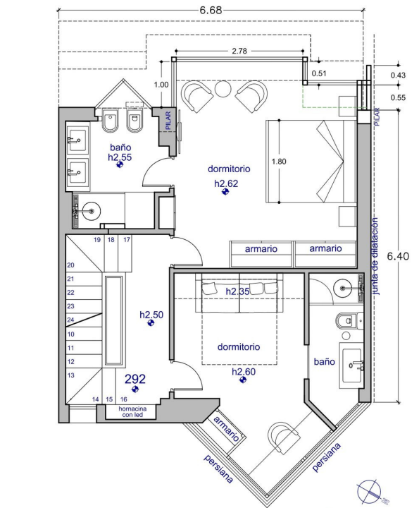
PLANTA SEGUNDA. 2 DORMITORIOS + 2 BAÑOS
