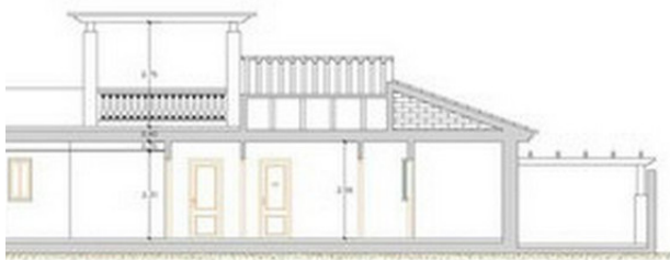
SECCION A-A
