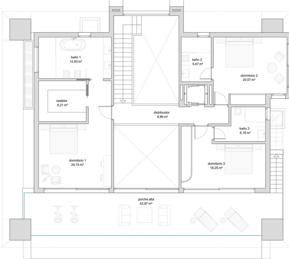
PLANTA ALTA
