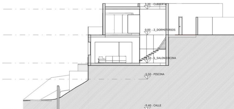
1 SECCIÓN ESCALERA A100
