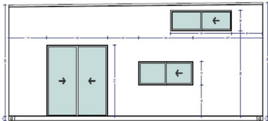
Alzado frontal
