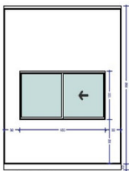
Alzado izquierdo
