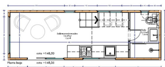
Planta baja
