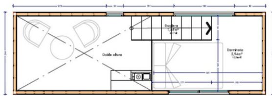
Planta alta
