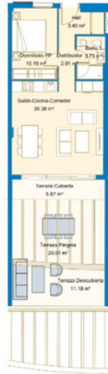
BLOQUE I_PLANTA PRIMERA_VIVIENDA 1.1.B 1:100
