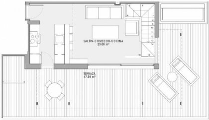
PLANTA ÁTICO
