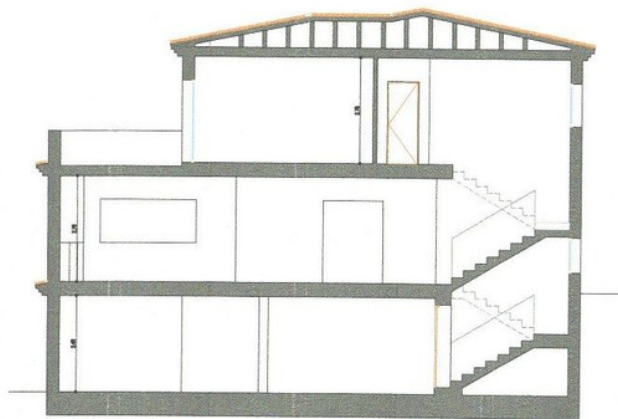
SECCION 1-1
