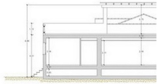
SECCION 8-8
