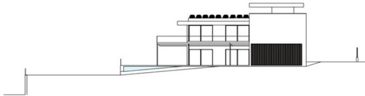
FACHADA NORESTE
