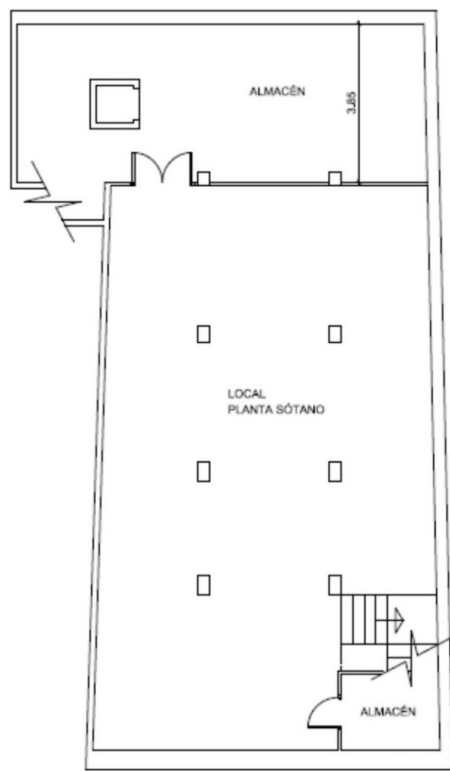
PLANTA SÓTANO
