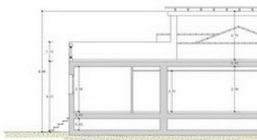
SECCION B-B
