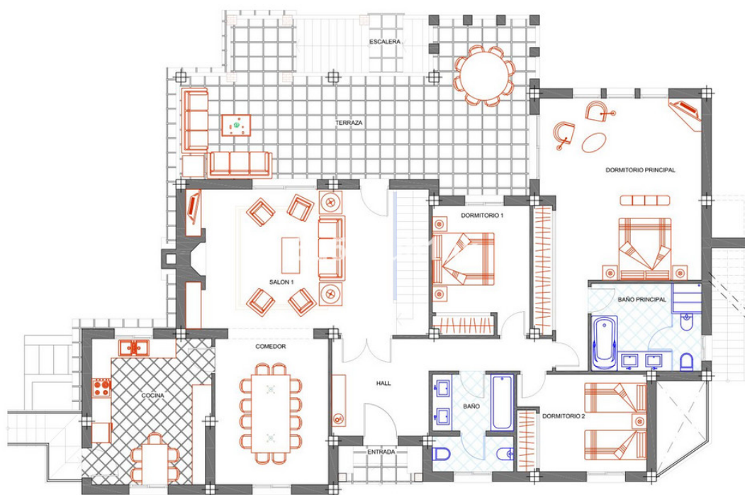
PLANTA ACCESO E=1/100
